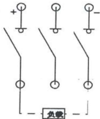
3P 外形接线图 (DC500V)
