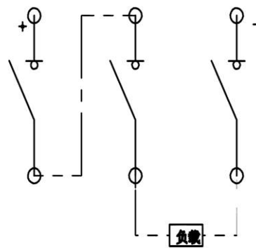
3P 外形接线图 (DC750V)
