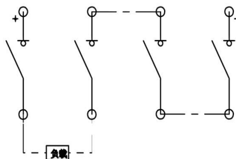
4P 外形接线图 (DC1000V)
